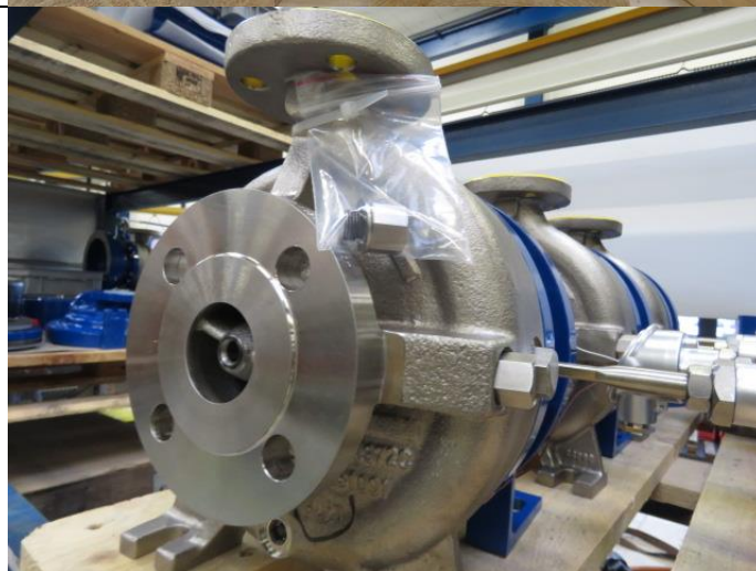
Bouchon de vidange MKP: démonté, mais attaché à la pompe.
