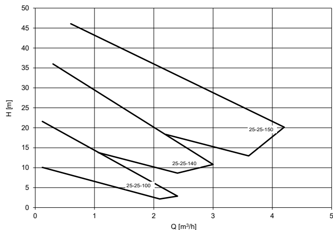
1800 min -1 /60 Hz
