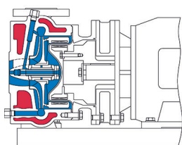
MKP Monoblock mit Heizung mit Grundplatte -100°C bis +250°C
