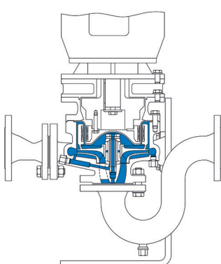
MKP Monoblock in-line vertikal mit Winkelständer -100°C bis +250°C
