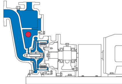
MKP-S Lagerstuhl mit Heizung (Heizpatrone) mit Grundplatte -100°C bis +250°C
