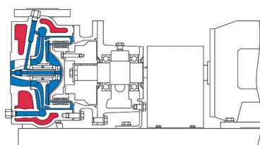
MKP Lagerstuhl mit Heizung mit Grundplatte -100°C bis +250°C
