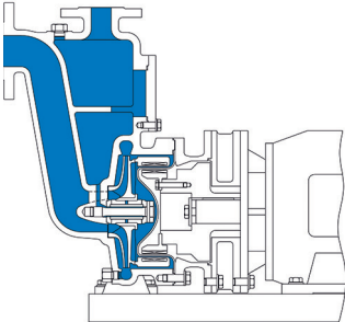
MKP-S Monoblock mit Grundplatte -100°C bis +250°C
