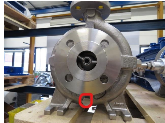
Bouchon de vidange MKP: monté (position normale)
