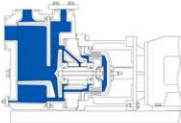
MKPL-S 一体式泵 带底板 -20 至 +150°C
