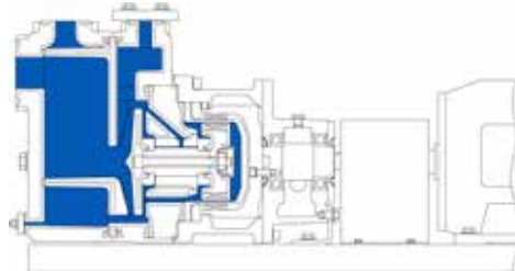
MKPL-S 轴承座式泵 带底板 -20 至 +150°C
