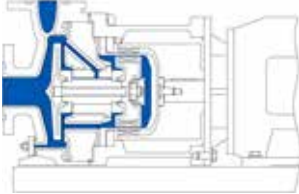
MKPL 一体式泵 带底板 -20 至 +200°C
