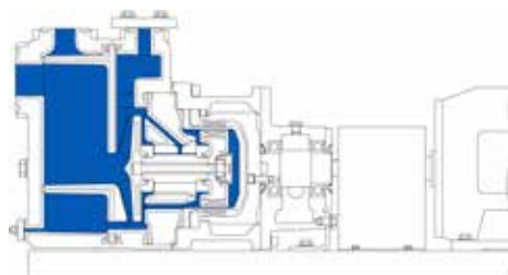
MKPL-S chaise palier avec plaque de base -20 à +150°C
