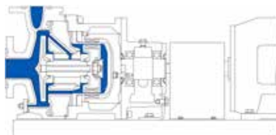
MKPL chaise palier avec plaque de base -20 à +200°C
