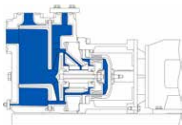
MKPL-S monobloc avec plaque de base -20 à +150°C
