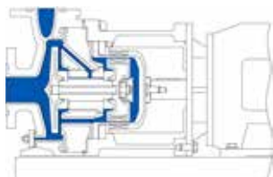
MKPL monobloc avec plaque de base -20 à +200°C
