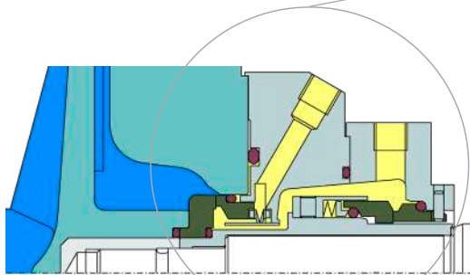
FuturaMik® Doppel-Gleitringdichtung
